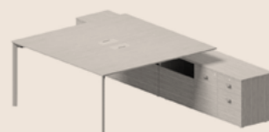
PORTE S1 K1614NKT / K1616NKT L: 1400-1673 / 1600-1873 mm D: 1600-2900 mm H: 740 mm
